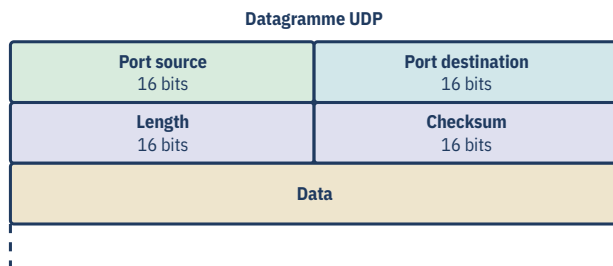
Fig. 53. – Format d'un datagramme UDP. Le champ «Length» indique la taille totale du datagramme, y compris l'en-tête. Le champ «Checksum» est utilisé pour vérifier l'intégrité des données. Les ports source et destination sont utilisés pour identifier les applications émettrices et destinataires.
